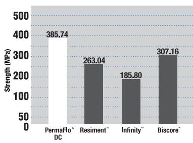
Druckfestigkeit; Wenn rein chemisch ausgehärtet, übertrifft PermaFlo DC andere namhafte Befestigungskomposite.
